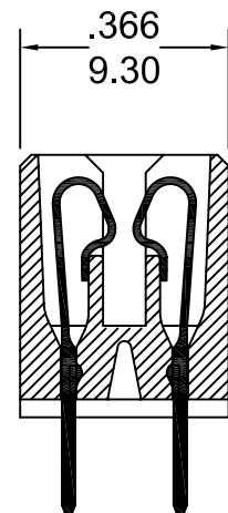
A-A SECTION
