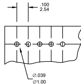
P.C.Board Hole Dimensions
