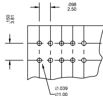
P.C.Board Hole Dimensions
